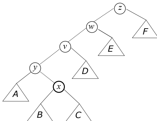
Figura 2: Mover a la raíz
