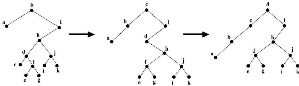
Figura 18: Casos extremos de acceso a un Splay. Luego de acceder al nodo b , accede al c y al d
