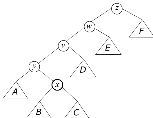
Figura 9: Se accede al nodo x en un árbol Splay
