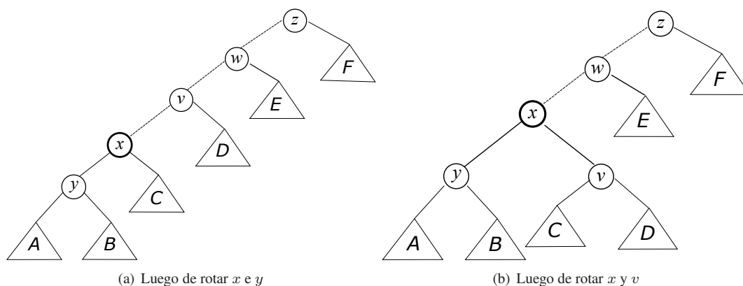
Figura 3: Mover x a la raíz
