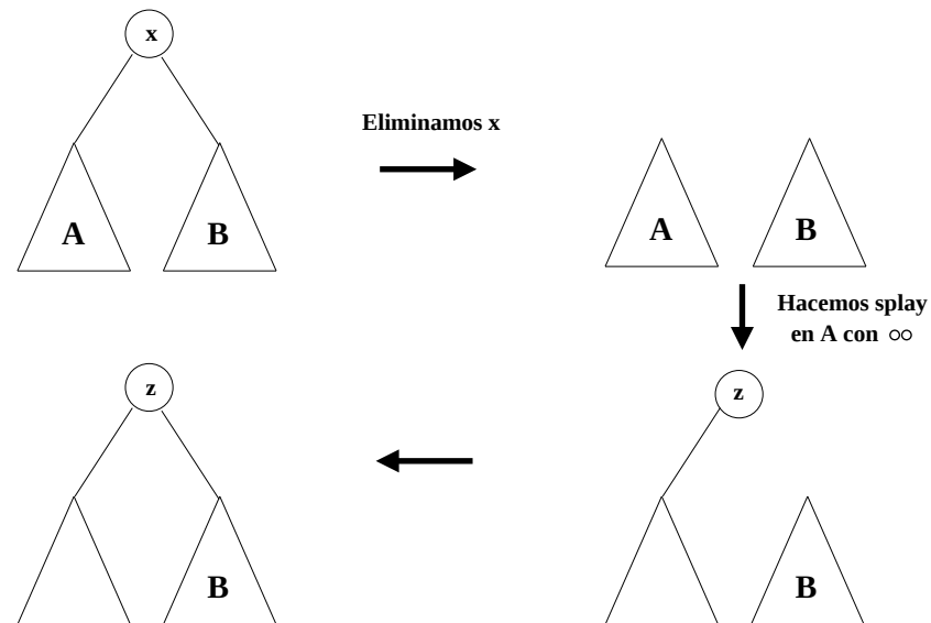
Figura 15: Modificación estructural necesaria para la eliminación del elemento x
