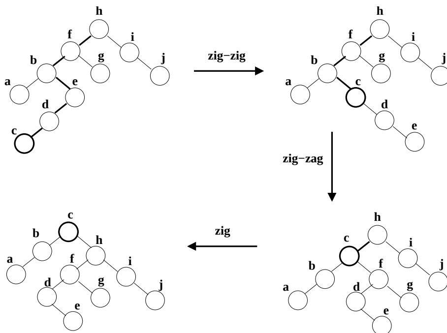
Figura 8: Ejemplo de splay sobre el nodo c
