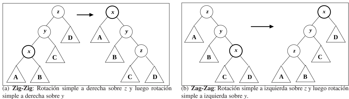
Figura 6: Zig-Zig y Zag-Zag , consisten en dos rotaciones simples a derecha o izquierda según corresponda
