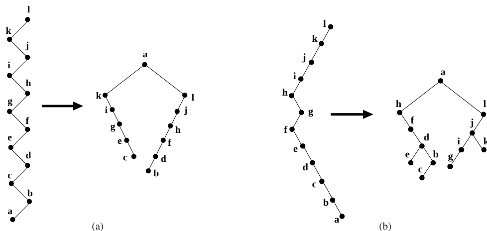
Figura 20: Casos de acceso extremo a un Splay desbalanceado
