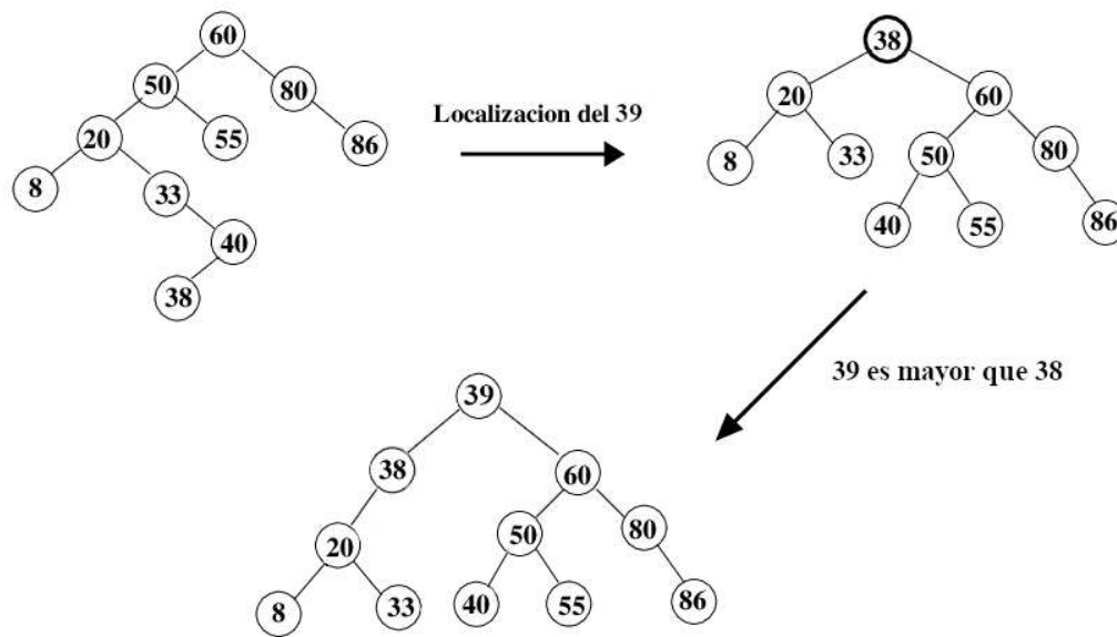
Figura 14: Inserción del elemento 39
