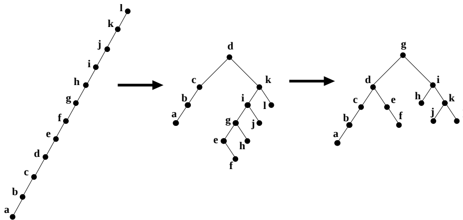
Figura 19: Casos costosos de acceso a un Splay; la secuencia es (d, g)
