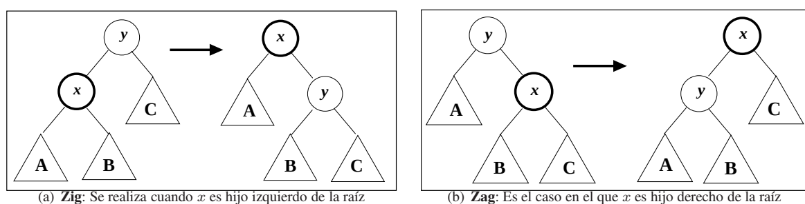
Figura 5: Zig y Zag , rotaciones simples y terminales
