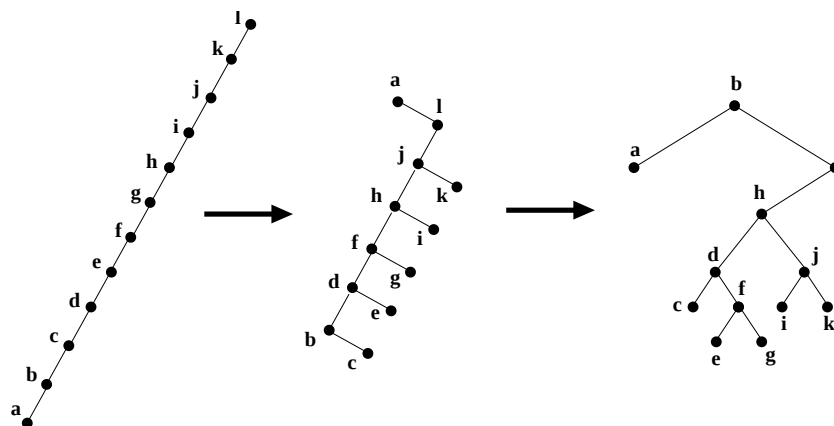
Figura 17: Casos extremos de acceso a un Splay . Primero se localiza el nodo a y luego el nodo b
