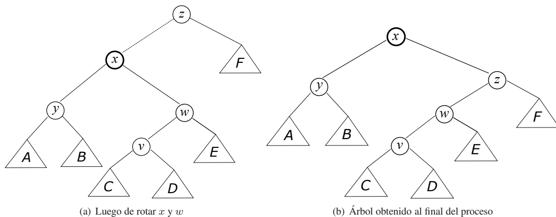
Figura 4: Mover x a la raíz
