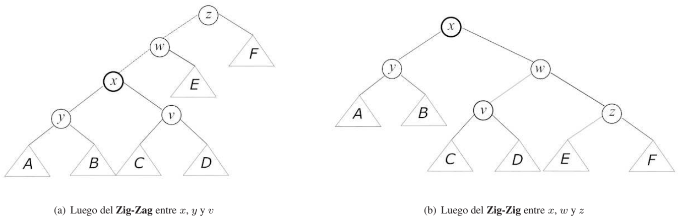
Figura 10: Proceso de splay luego de acceder al nodo x
