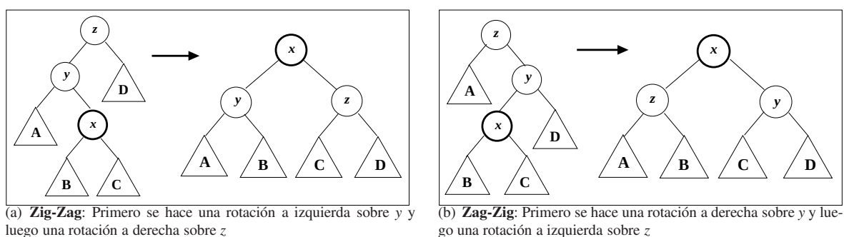
Figura 7: Zig-Zag y Zag-Zig , consisten en una rotación doble a derecha o izquierda según corresponda
