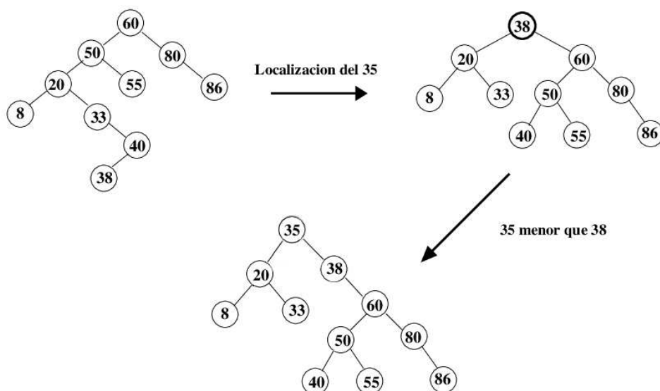
Figura 13: Inserción del elemento 35
