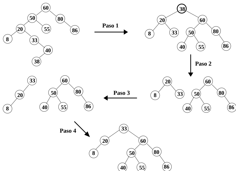
Figura 16: Eliminación del elemento 38
