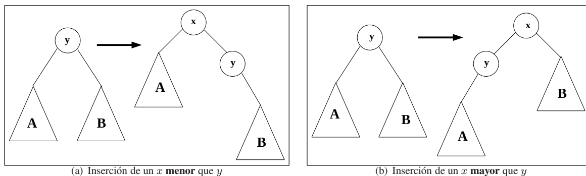
Figura 12: Modificación estructural del Splay durante una inserción
