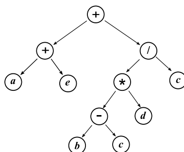
Figura 3: (a + e + (b - c) * d/c)
