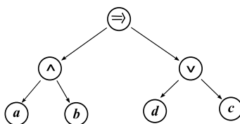
Figura 1: Árbol de expresión para (a \wedge b) \Rightarrow (d \vee c)
